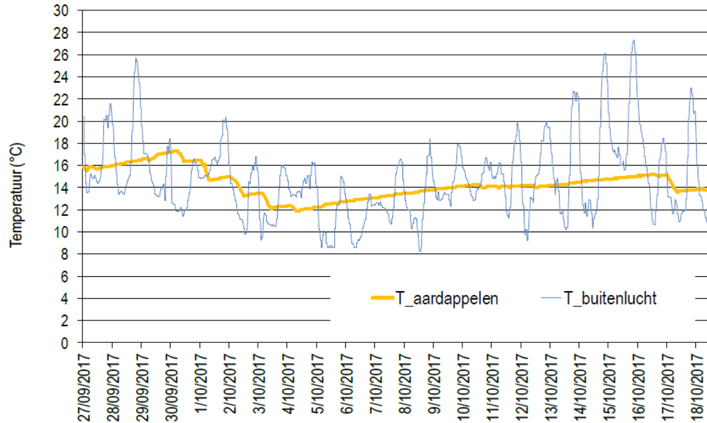
Temperatuurverloop in een aardappelloods
